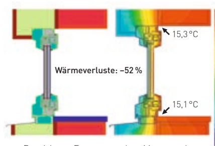
>> Passivhaus-Fenster vor dem Mauerwerk
