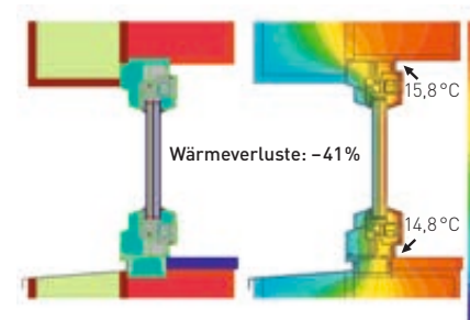
>> Passivhaus-Fenster bündig zum Mauerwerk
