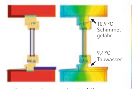
>> Typischer Fenstereinbau im Altbau
