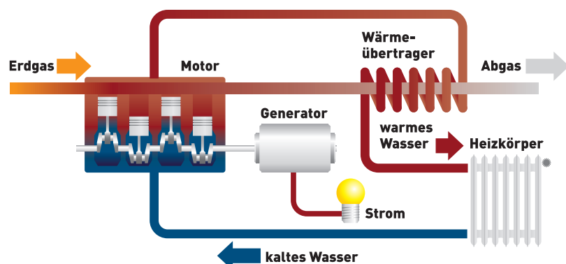
Prinzip des BHKW
