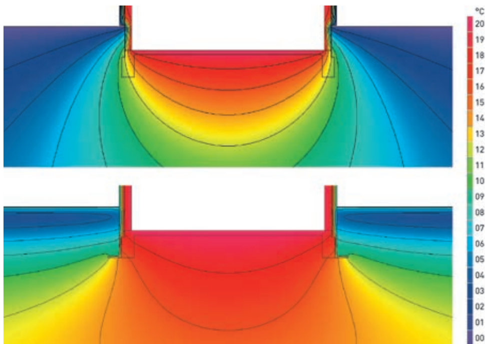
Temperaturverlauf Anfang Januar bei einem Schnitt durch einen Keller und das umliegende Erdreich. Oben ohne Dämmschürze und unten mit Dämmschürze. Deutlich zu erkennen sind die höheren Temperaturen der Kellerwände und des Erdreichs unter dem Keller bei der Variante mit Dämmschürze.
